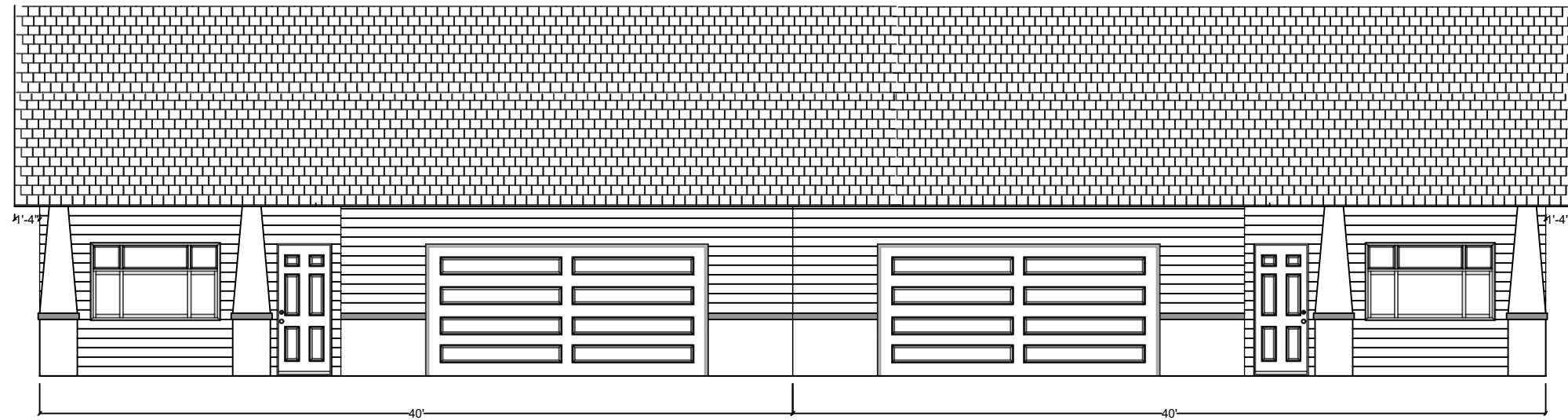
D 1 ELEVATION SCALE: 1/8" = 1'-0"
